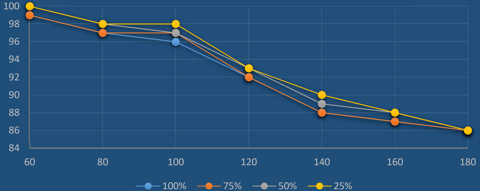
Return Water Temperature (°F)
