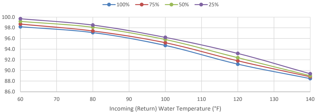
SONIC SC-2000 Thermal Efficiencies @ 60°F ΔT
